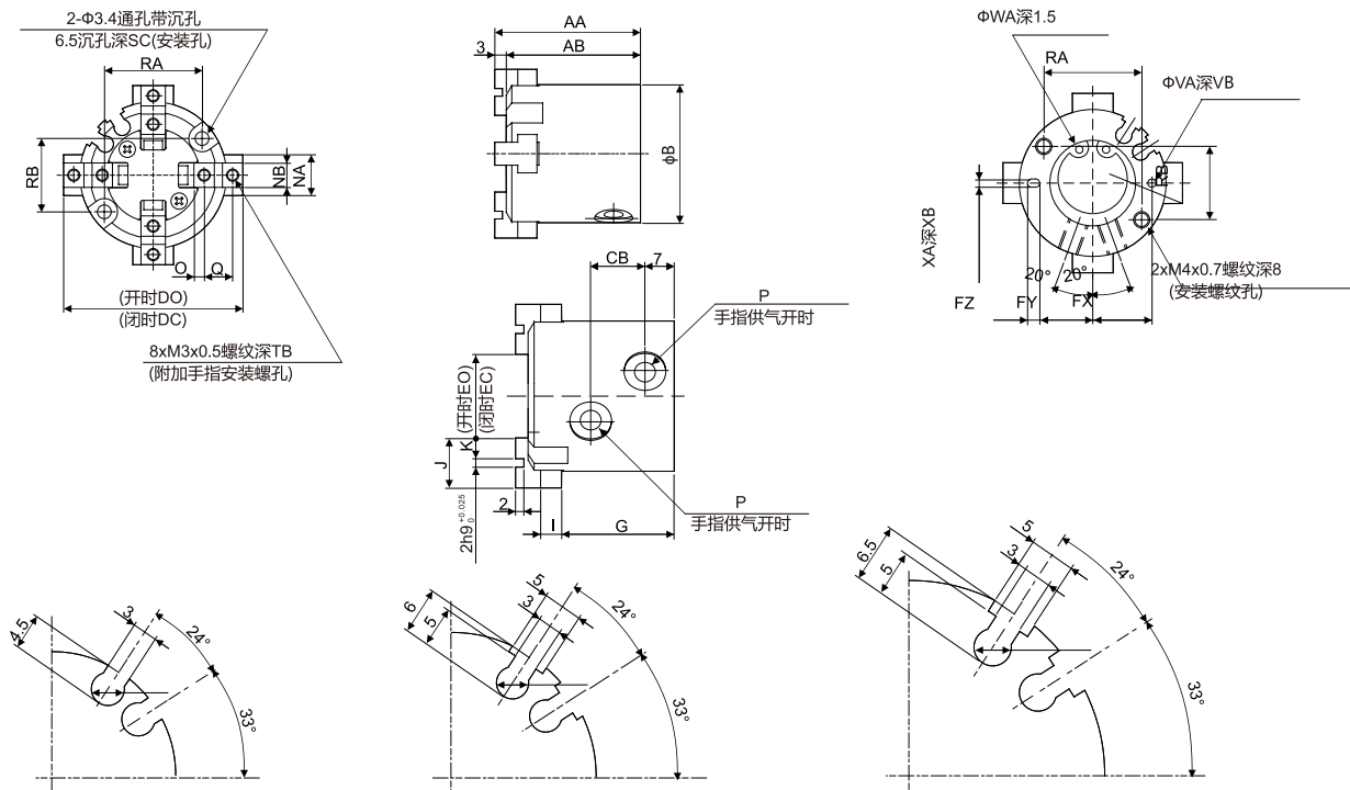
NMHS4-□ Φ16D/Φ25D
