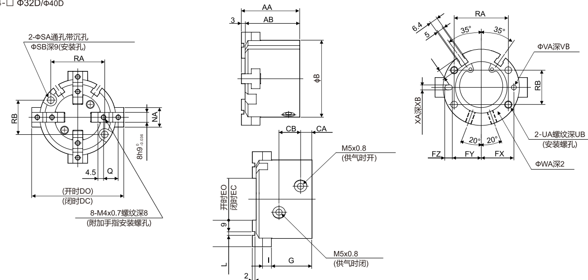
NMHS4-□ Φ32D/Φ40D
